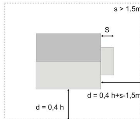
Constructions - vue en plan
